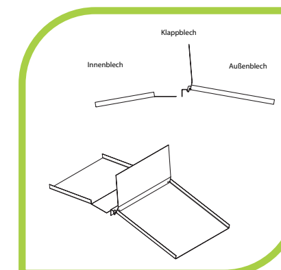
Tür auf; Klappblech fixiert, zweiteilig
